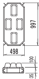
大型覆土ブロック半丁H135
