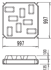
大型覆土ブロック半丁H135
