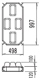
大型覆土ブロック半丁H120
