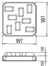
大型覆土ブロック半丁H150
