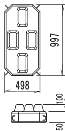
大型覆土ブロック半丁H150
