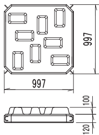
大型覆土ブロック半丁H120
